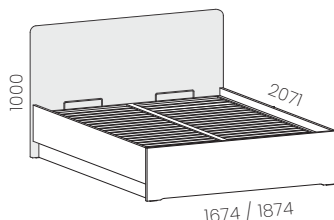
ML 160DT / 200 ML 180DT / 200
