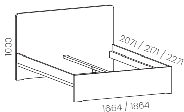
ML 160V / 200 1 , 210 2 , 220 2 ML 180V / 200 3 , 210 3 , 220 3
