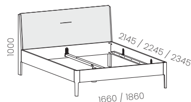
ML 160KT / 200 4 , 210 4 , 220 4 ML 180KT / 200 4 , 210 4 , 220 4
