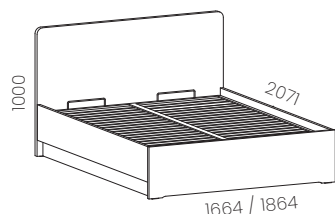
ML 160D / 200 ML 180D / 200
